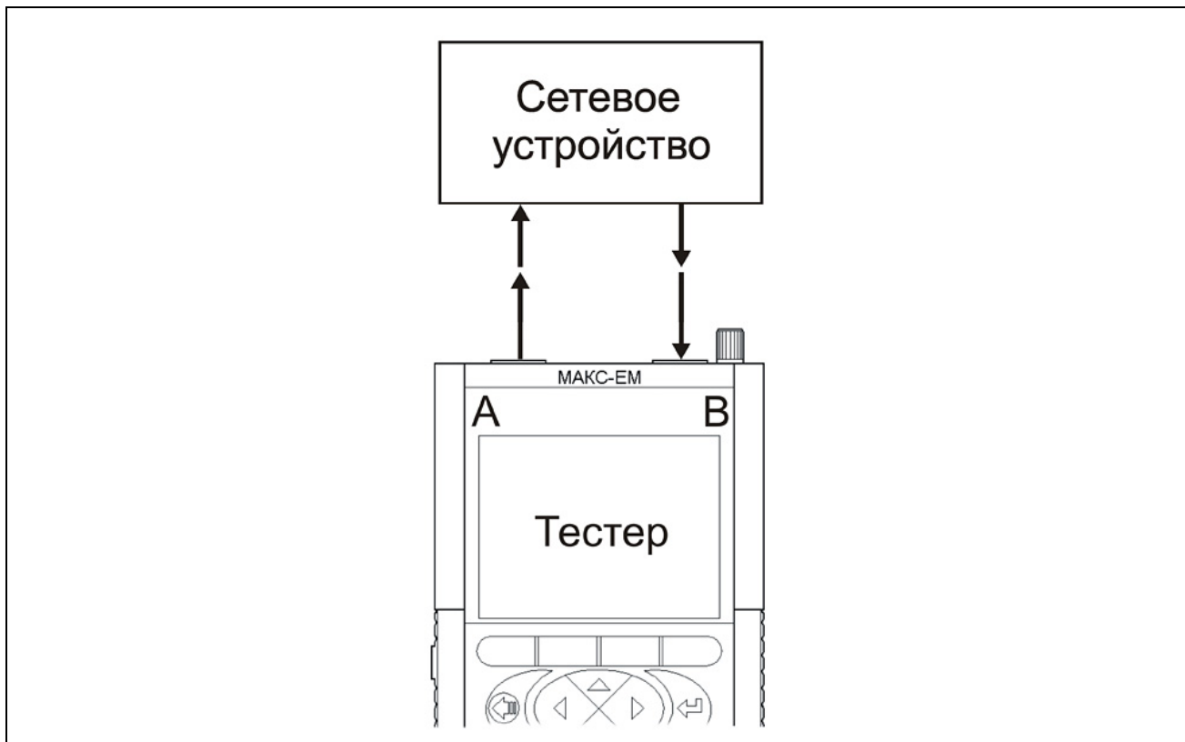
Рисунок 10.4.2. Схема «В» подключения прибора в режиме тестирования
