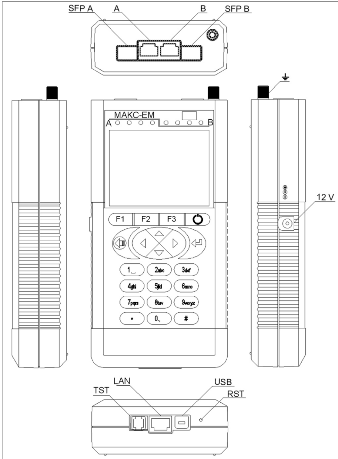
Рисунок 4.1.4. Схема расположения разъемов прибора
