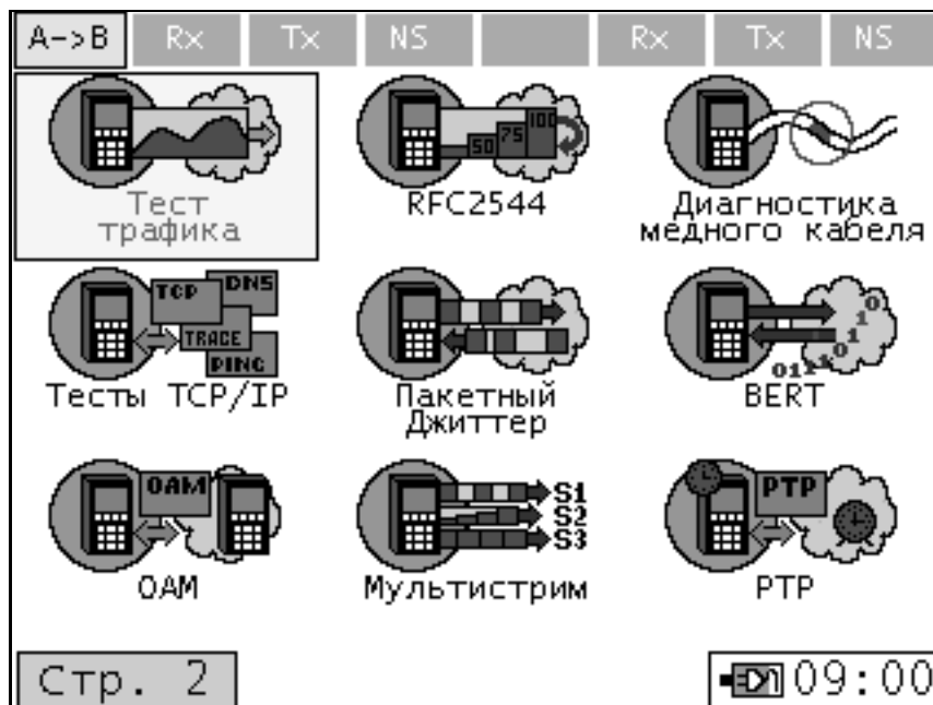
Рисунок 10.3.1. Первая страница меню «Измерения»
