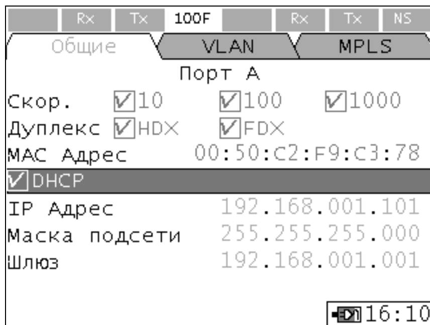
Рисунок 10.19.2. Параметры интерфейсов. Общие
