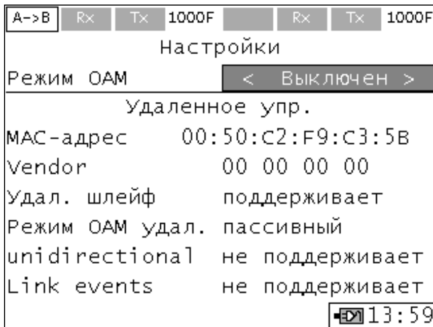
Рисунок 10.13. Удаленное управление OAM
