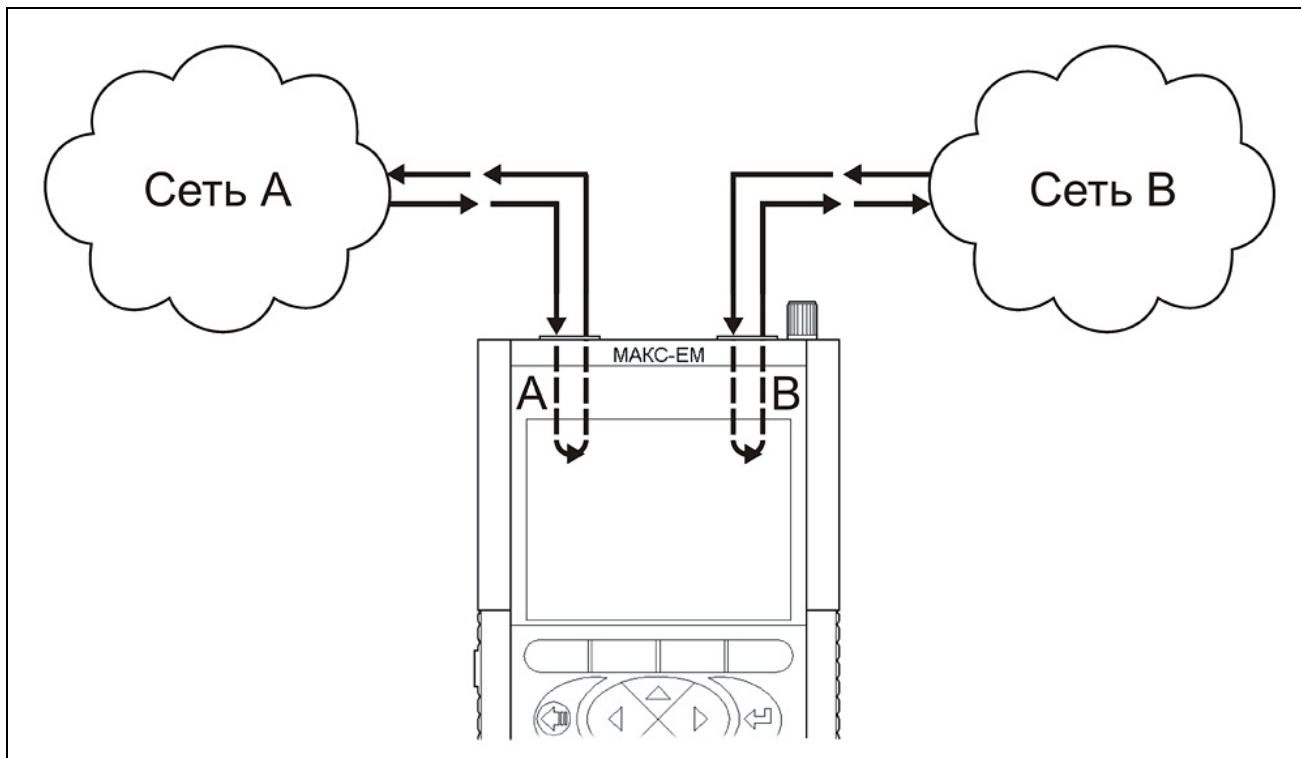
Рисунок 10.15. Схема подключения в режиме Шлейф
