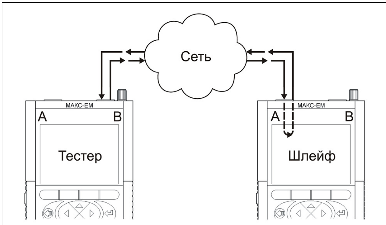
Рисунок 10.4.1. Схема «А» подключения прибора в режиме тестирования
