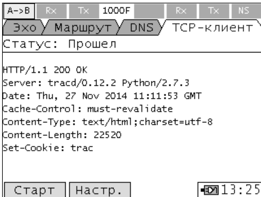
Рисунок 10.11.4. TCP - клиент
