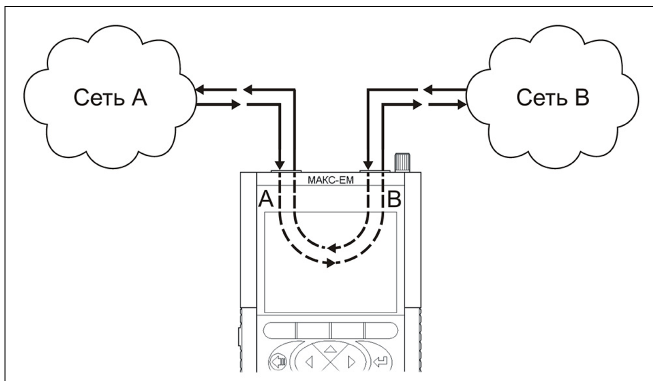
Рисунок 10.16. Схема подключения в режиме Транзит
